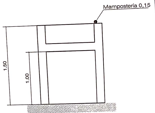
VISTA ESC 1:75
