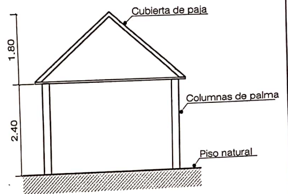
VISTA ESC 1:100
